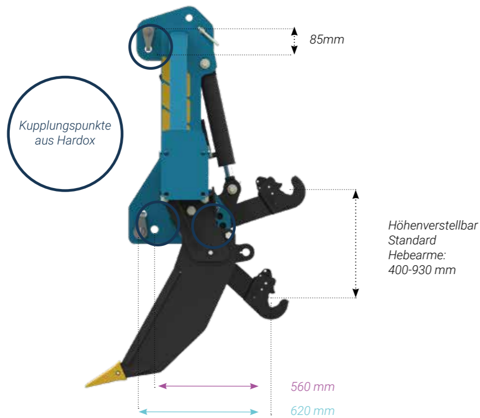
Illustration des kurzen Anbauraums des Tiefenlockerers Culter
